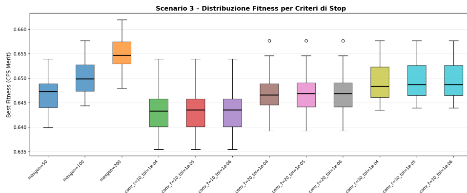
Figura 40: Fitness boxplot per lo scenario criteri di stop
