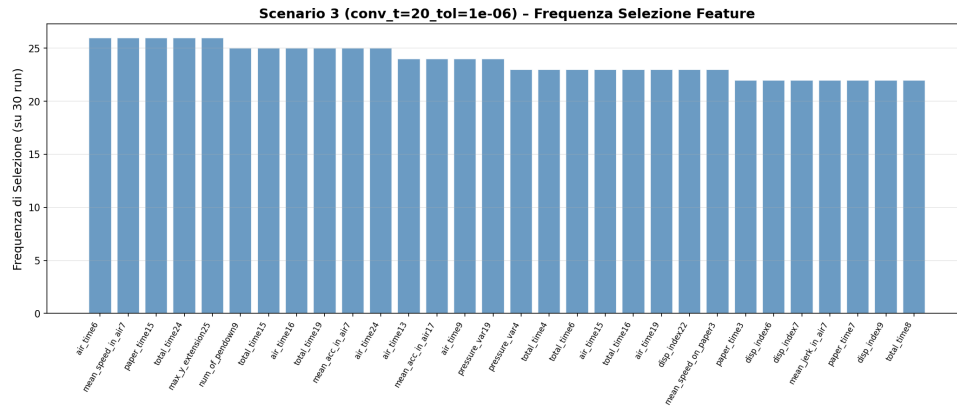
Figura 36: Frequenza di selezione delle feature per lo scenario criteri di stop-finestra di convergenza 20-tolleranza 1e-06
