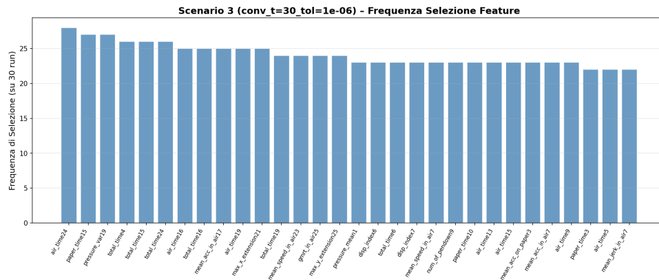
Figura 39: Frequenza di selezione delle feature per lo scenario criteri di stop-finestra di convergenza 30-tolleranza 1e-06
