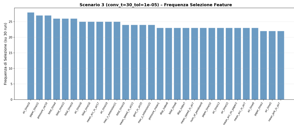
Figura 38: Frequenza di selezione delle feature per lo scenario criteri di stop-finestra di convergenza 30-tolleranza 1e-05
