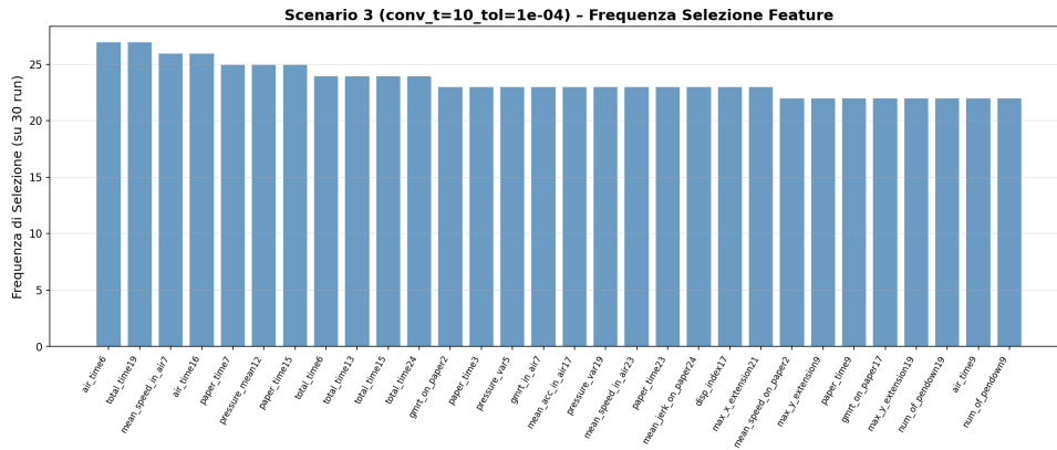
Figura 31: Frequenza di selezione delle feature per lo scenario criteri di stop-finestra di convergenza 10-tolleranza 1e-04
