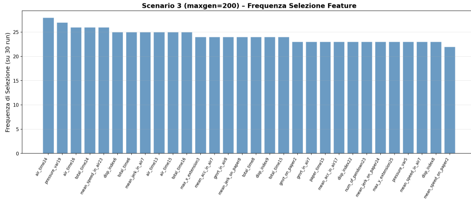
Figura 30: Frequenza di selezione delle feature per lo scenario criteri di stop-numero di generazioni fisso 200
