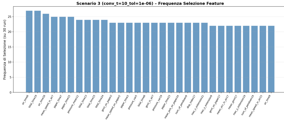
Figura 33: Frequenza di selezione delle feature per lo scenario criteri di stop-finestra di convergenza 10-tolleranza 1e-06
