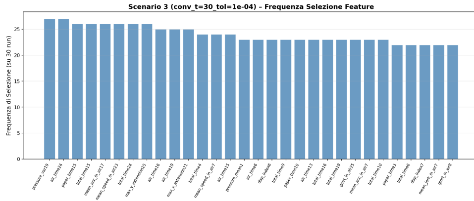
Figura 37: Frequenza di selezione delle feature per lo scenario criteri di stop-finestra di convergenza 30-tolleranza 1e-04
