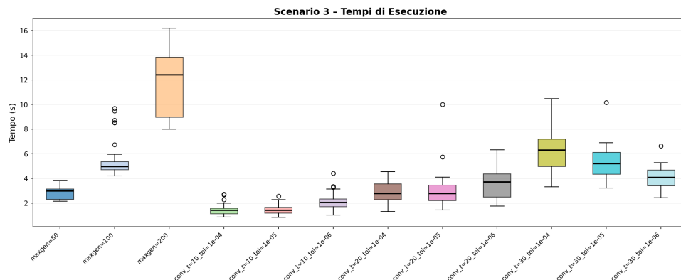
Figura 27: Tempo di esecuzione per lo scenario criteri di stop
