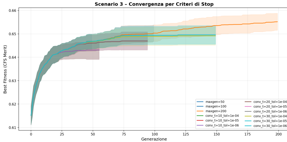
Figura 26: Convergenza per lo scenario criteri di stop
