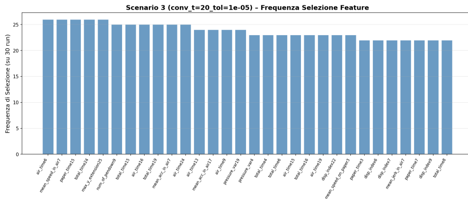
Figura 35: Frequenza di selezione delle feature per lo scenario criteri di stop-finestra di convergenza 20-tolleranza 1e-05
